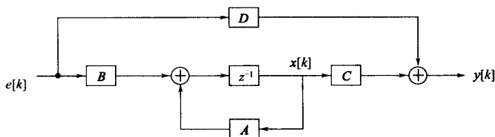
图 9-18 离散系统状态变量分析的示意图
