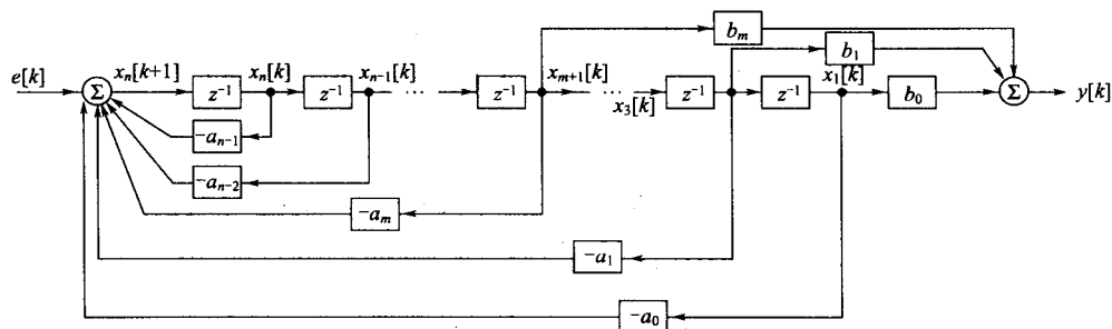
图 9-19 离散系统的可控规范型实现
