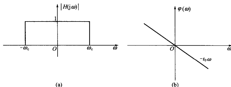
图 3-30 理想低通滤波器特性
