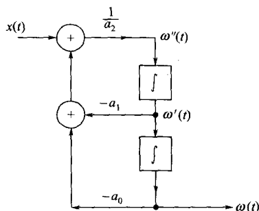
图 2-26 式(2-94) 所描述系统的模拟框图
