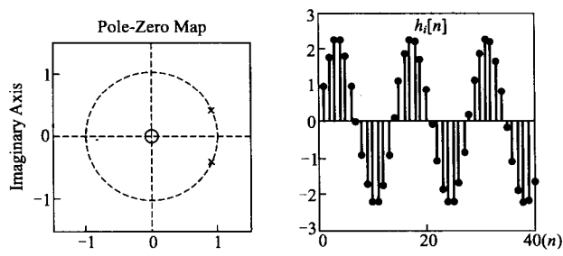
图 8-7 单位圆上一阶共轭极点及其对应的时间信号
