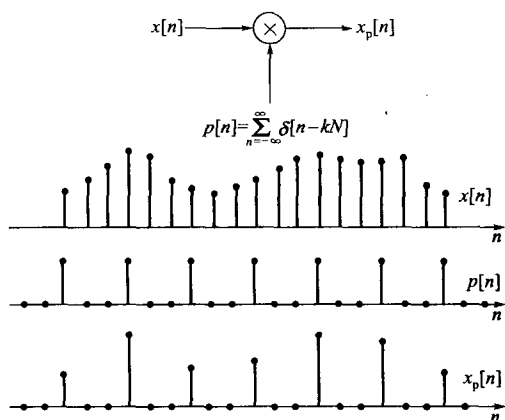
图 5-15 离散时间脉冲串采样
