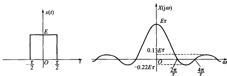
图 3-15 矩形窗函数的波形、频谱
