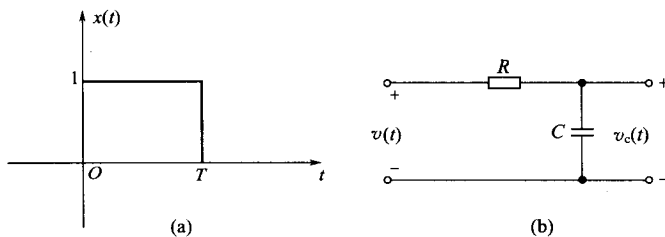
图 3-34 RC 低通网络
