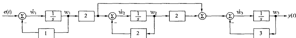
图 9-13 串联实现
