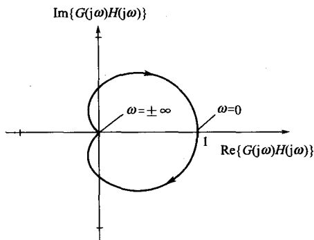
图 8-38 例 8-14 的 G(j\omega)H(j\omega) 的奈奎斯特图
