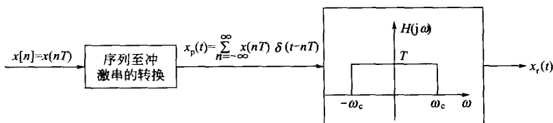
图 5-4 恢复系统
