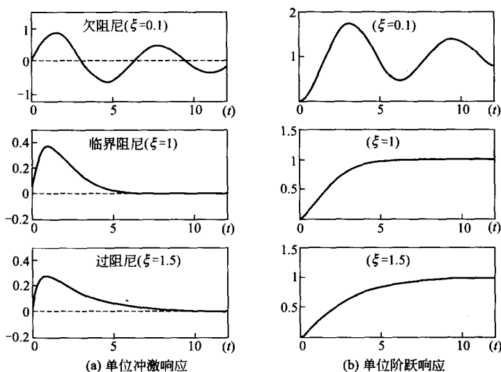
图 8-14 不同阻尼系数下的二阶系统响应
