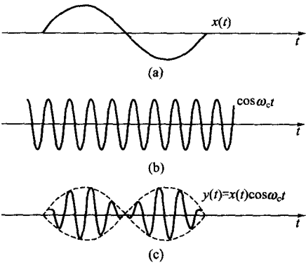
图 5-32 DSB 调制波形
