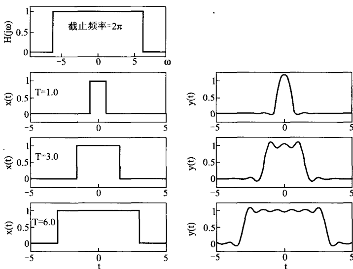
图 3-33 理想低通滤波器对矩形脉冲的响应
