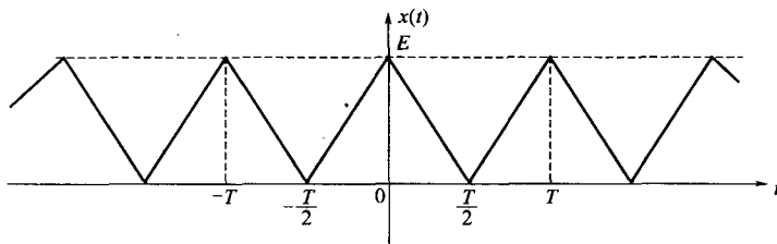
图 3-5 周期三角脉冲信号的波形
