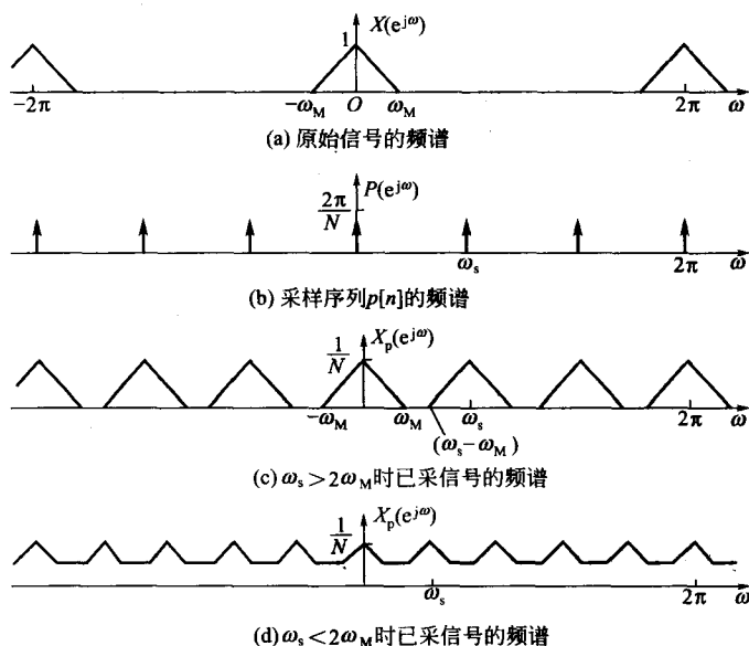
图 5-16 脉冲串采样后的频谱图
