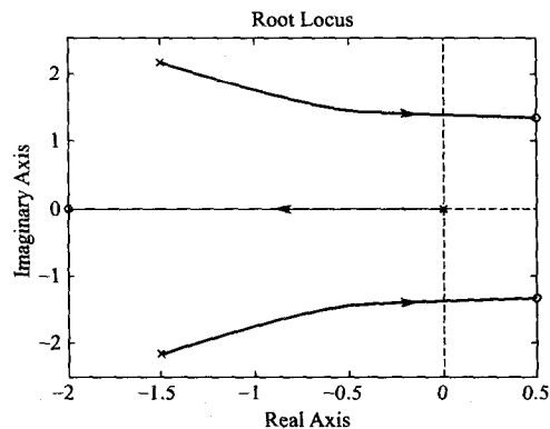
图 8-44 例 8-20 的根轨迹
