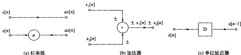
图 2-29 离散系统的三个基本运算单元
