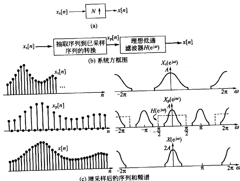
图 5-20 信号的增采样 (内插)
