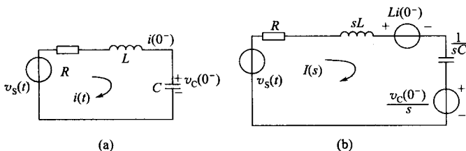
图 6-25 RLC 电路 S 域模型
