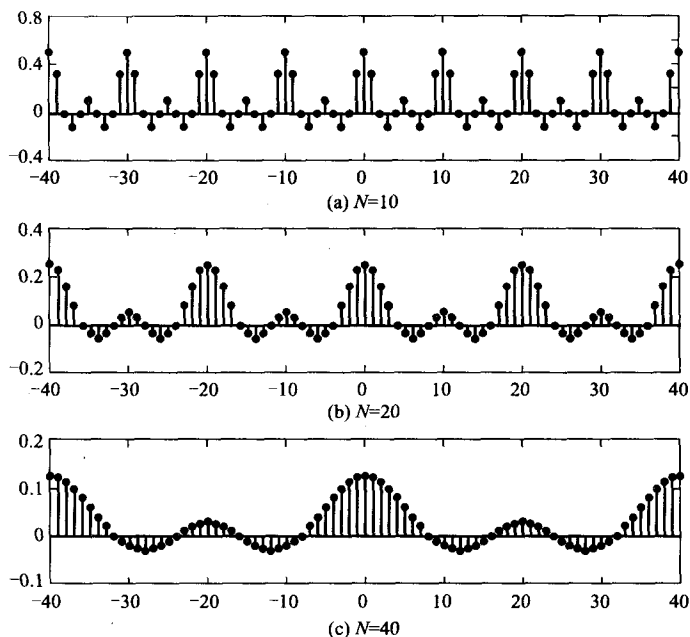
图 4-2 例 4-2 周期方波的傅里叶级数系数
