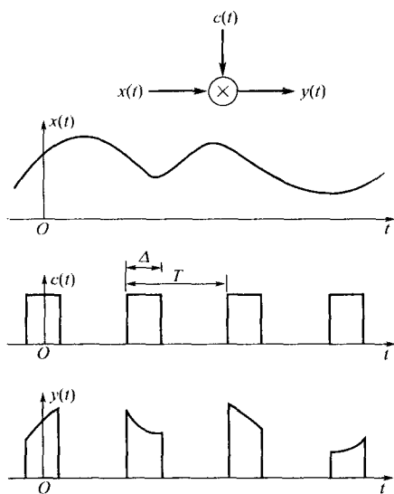
图 5-38 自然采样形式的脉冲幅度调制
