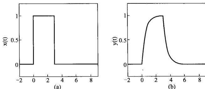
图 3-27 RC 低通网络对矩形脉冲的响应, E=1.0 , T=3.0
