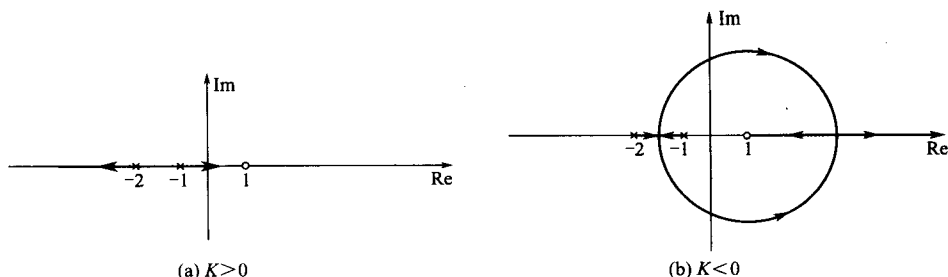
图 8-30 例 8-10 的根轨迹
