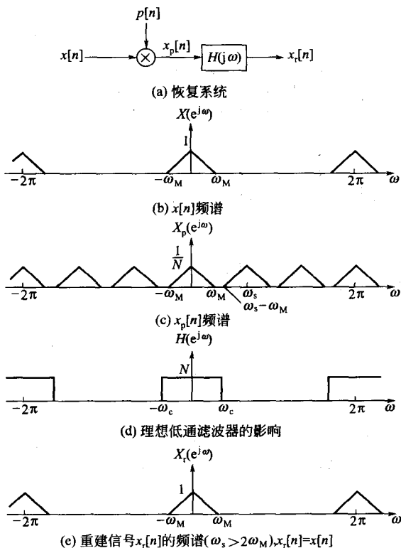
图 5-17 从样本中精确重建 x[n] 的恢复系统
