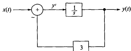
图 6-28 例 6-23 S 域模拟框图
