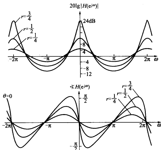
图 8-18 由方程式(8-65)所描述的二阶系统的幅频响应与相频响应
