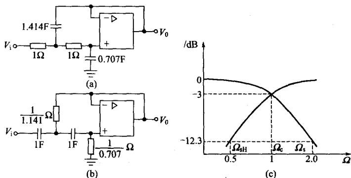
图 8-24 低通与高通滤波器的幅频特性
