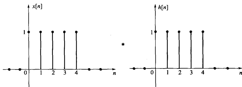
图 2-18 例 2-7 中 x[n] 和 h[n] 的波形
