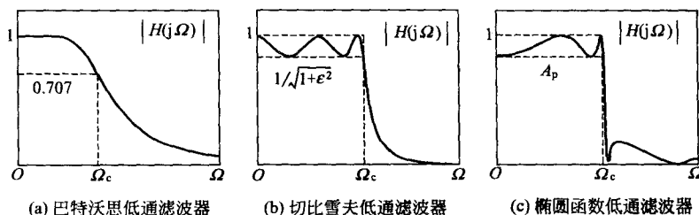
图 8-20 三种常用的低通滤波器的幅频特性
