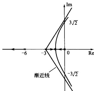
图 8-33 例 8-12 的根轨迹
