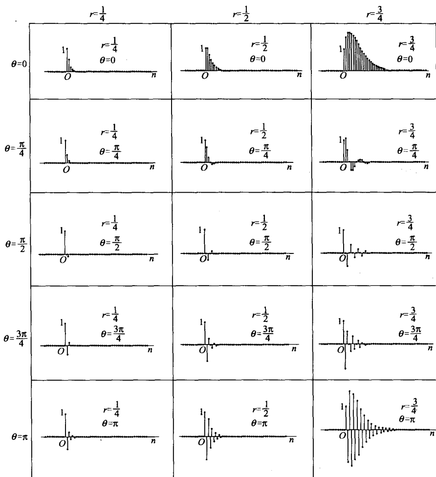
图 8-16 由方程式(8-65)表示的二阶系统的单位脉冲响应
