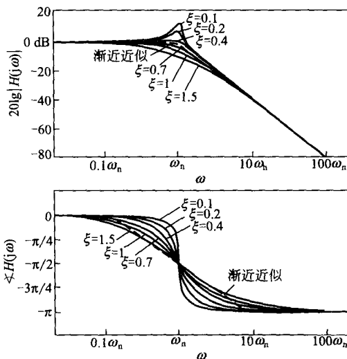
图 8-15 不同阻尼系数 \xi 值下, 二阶系统的波特图
