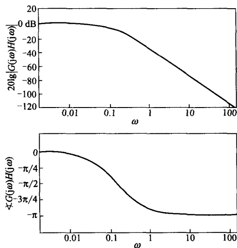
图 8-37 例 8-14 的 G(j\omega)H(j\omega) 的波特图
