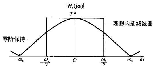
图 5-8 零阶保持和理想滤波器的频响特性
