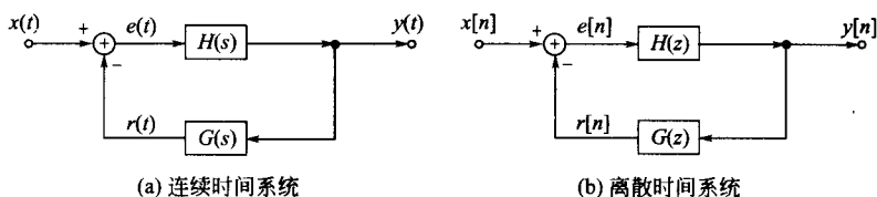
图 8-25 基本 LTI 反馈系统结构
