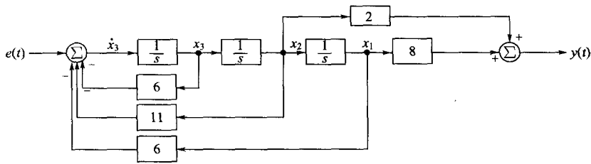
图 9-15 可控规范型实现
