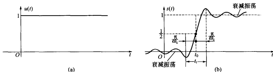
图 3-32 理想低通滤波器的阶跃响应
