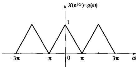
图 4-16 x[n] = \frac{1}{2} \text{Sa}^2\left(\frac{\pi n}{2}\right) 的傅里叶变换
