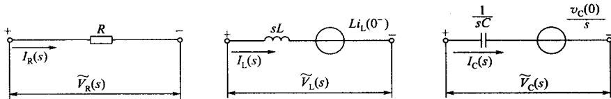
图 6-23 元件的电压降与电流关系的 S 域模型 (回路分析)
