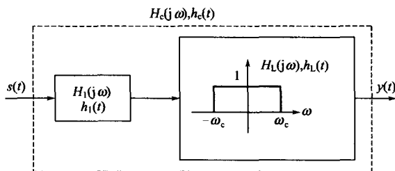
图 5-29 带限回波消除器
