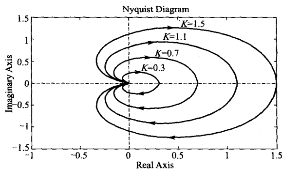
图 8-43 例 8-19 的奈奎斯特图
