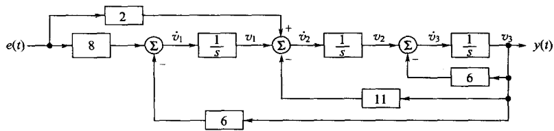
图 9-16 可观规范型
