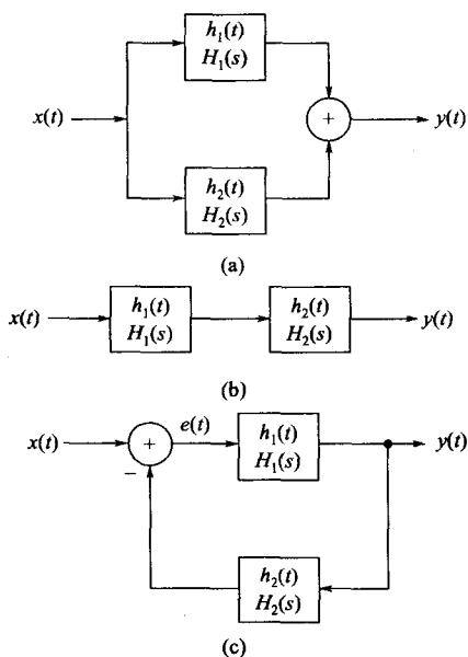
图 6-26 系统基本的连接方框图
