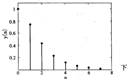
图 7-13 例 7-29 零状态响应波形
