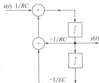
图 2-38 LC 并联电路的模拟框图
