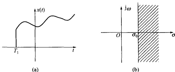
图 6-7 右边信号及其收敛域
