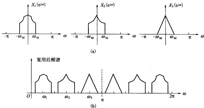
图 5-47 离散时间频分复用系统中的有关频谱 (3 路)
