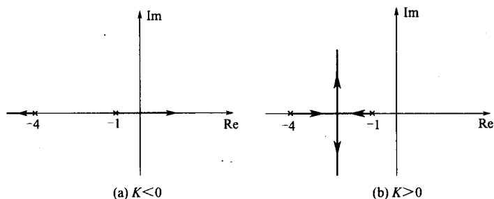
图 8-28 例 8-9 的根轨迹
