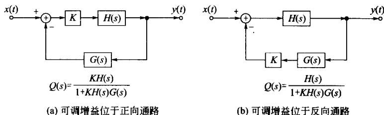
图 8-26 包含一个可调增益的反馈系统
