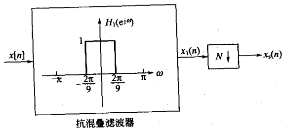
图 5-21 信号的最大抽取
