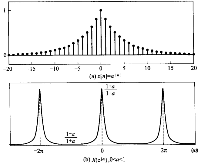
图 4-6 双边指数衰减信号及其频谱
