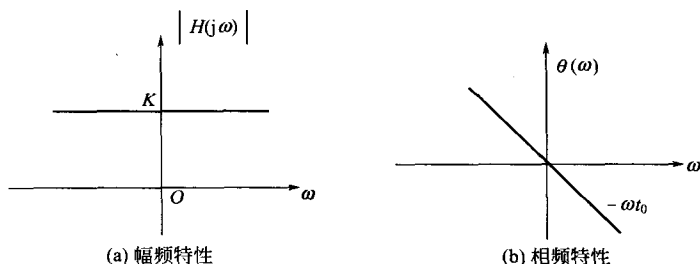
图 3-28 无失真传输系统的频率响应特性
