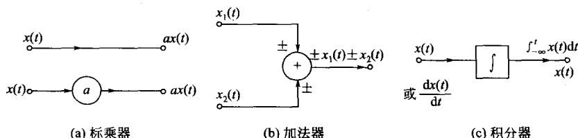
图 2-25 三种基本运算器的模型符号
