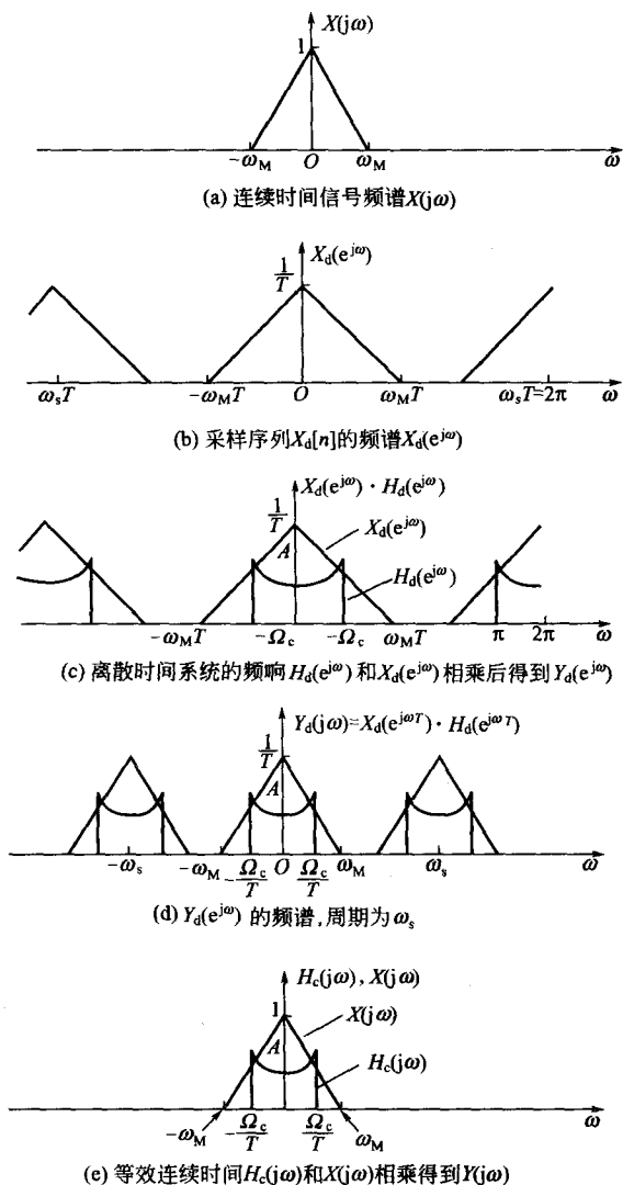
图 5-27 系统的频域说明
