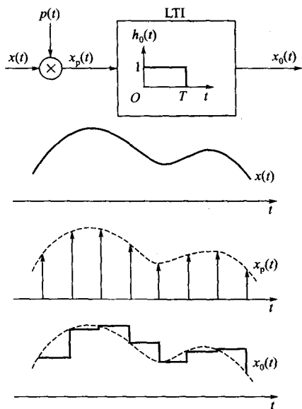
图 5-13 零阶保持采样的数学模型
