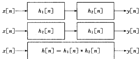
图 2-20 离散时间 LTI 系统的级联
