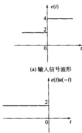
(a) 输入信号波形 (b) t < 0 时输入信号波形 图 2-24 例 2-17 的 输入信号波形
