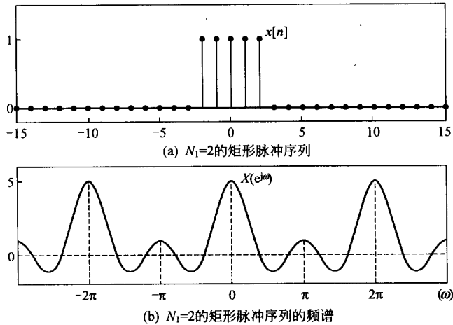
图 4-7 矩形脉冲序列及其频谱
