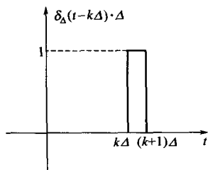
图 2-3 \delta_{\Delta}(t-k\Delta) \cdot \Delta 的波形
