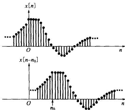
图 1-51 离散信号的平移
