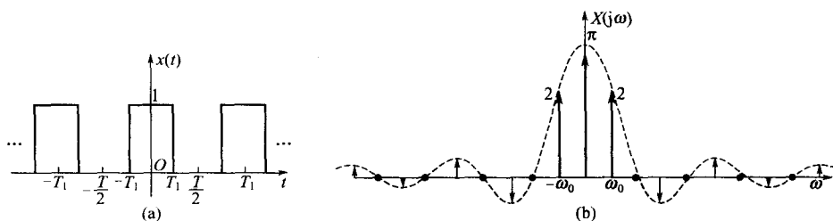
图 3-18 周期对称方波的傅里叶变换 ( T=4T_1 )
