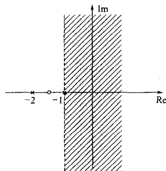
图 6-4 例 6-3 的收敛域
