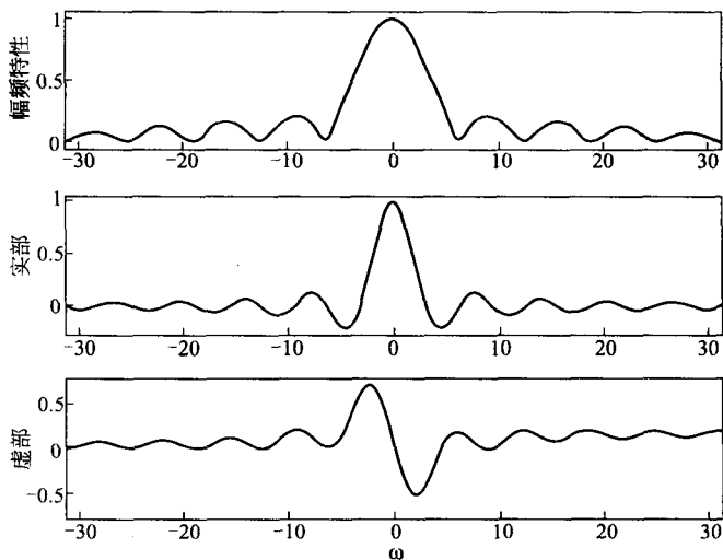
图 3-17 方波的频谱
