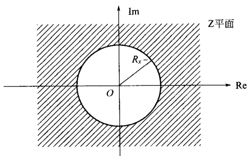
图 7-3 右边序列的 ROC
