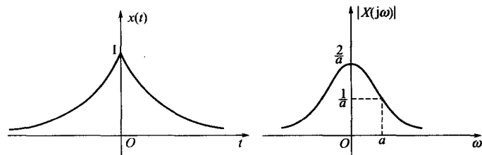
图 3-12 双边指数信号的波形及频谱
