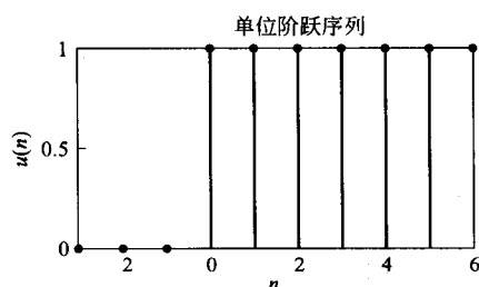
图 1-37 单位阶跃序列波形 (例 1-6 图)
