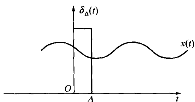
图 1-27 x(t) 与 \delta_\Delta(t) 的乘积
