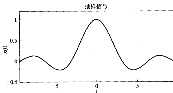
图 1-32 抽样信号 (例 1-4 图)
