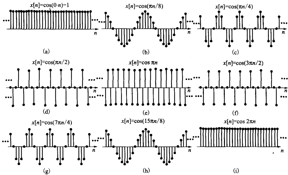
图 1-43 \omega_0 变化时的正弦序列
