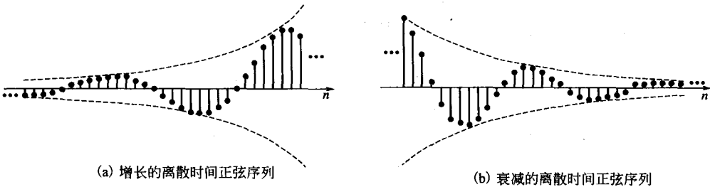
图 1-44 衰减的正弦序列和增长的正弦序列
