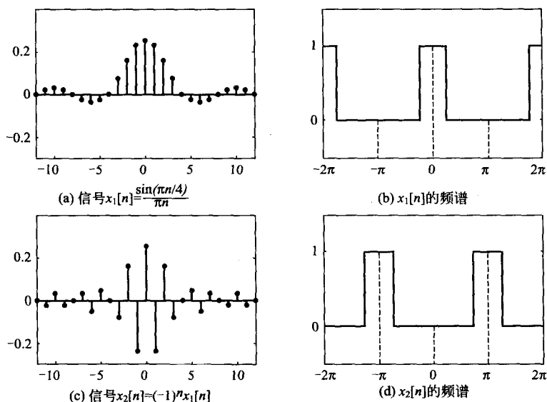
图 4-4 离散时间低频信号与高频信号的频谱
