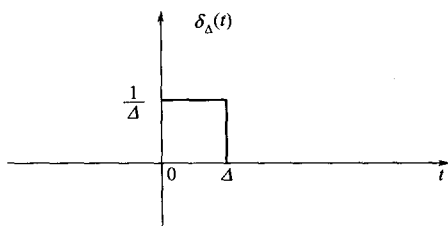
图 1-25 \delta_\Delta(t) 的波形
