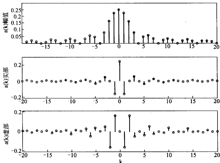
图 3-7 占空比为 25% 的非对称周期方波的傅里叶级数的系数
