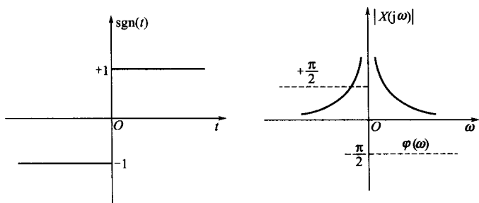
图 3-22 符号函数波形和频谱
