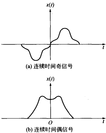
图 1-6 连续时间奇信号与偶信号
