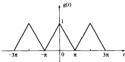
图 4-15 周期三角脉冲信号
