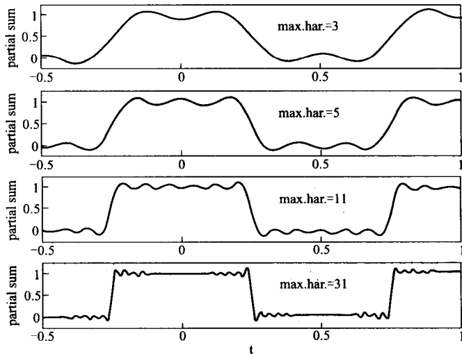
(a) 用有限项谐波叠加近似表示占空比为 0.5 的方波
