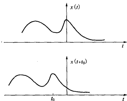
图 1-50 连续时间信号的平移
