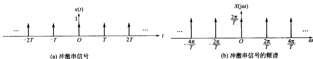
图 3-20 冲激串频谱
