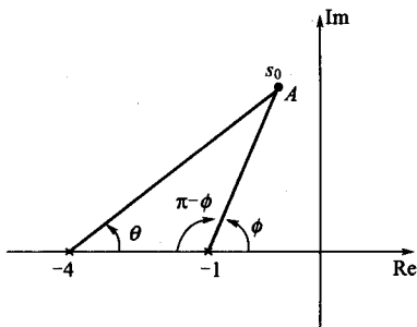
图 8-27 求满足角判据的几何方法
