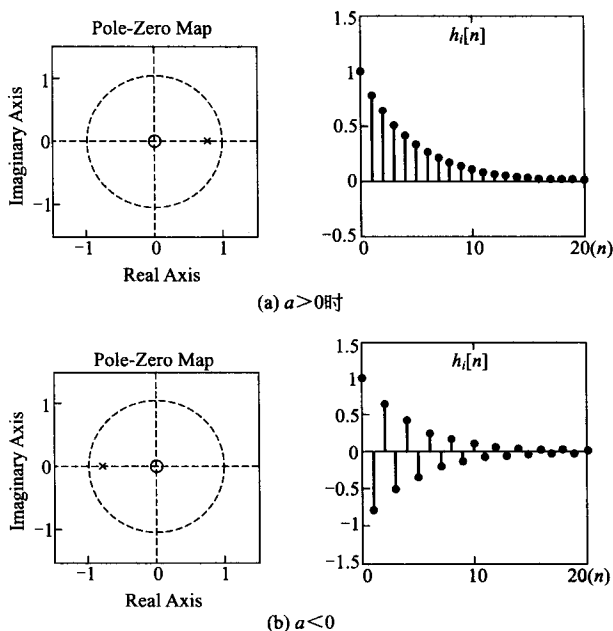
图 8-3 单位圆的一阶实极点及其对应的时间信号
