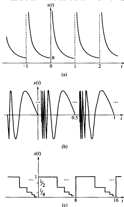
图 3-8 不满足狄里赫利条件的信号
