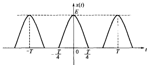
图 3-6 周期半波余弦信号波形
