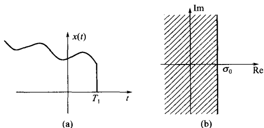
图 6-8 左边信号及其收敛域
