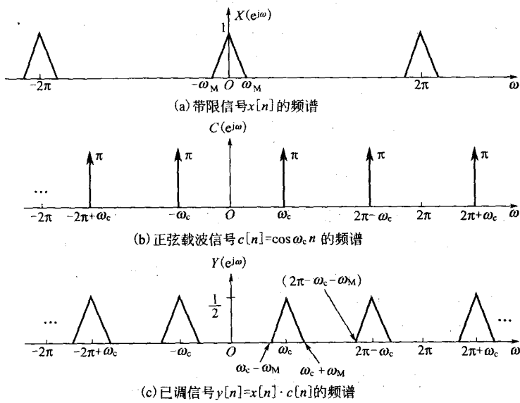
图 5-45 正弦载波的离散时间幅度调制的频谱说明
