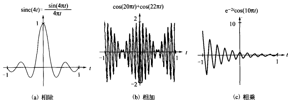
图 1-45 信号的组合
