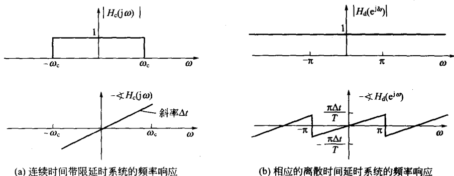
图 5-30 带限延时器的频率响应
