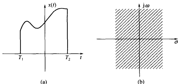
图 6-5 时限信号 x(t) 及其收敛域
