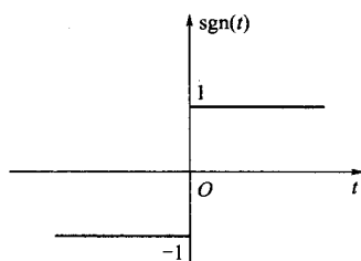
图 1-23 符号函数 \text{sgn}(t)
