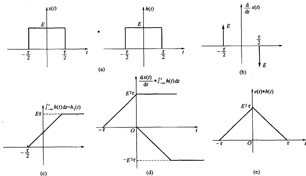
图 2-16 用卷积微分、积分性质计算卷积
