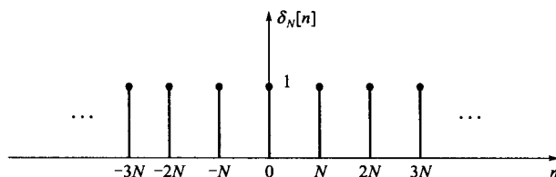
图 1-40 单位离散冲激串序列的波形
