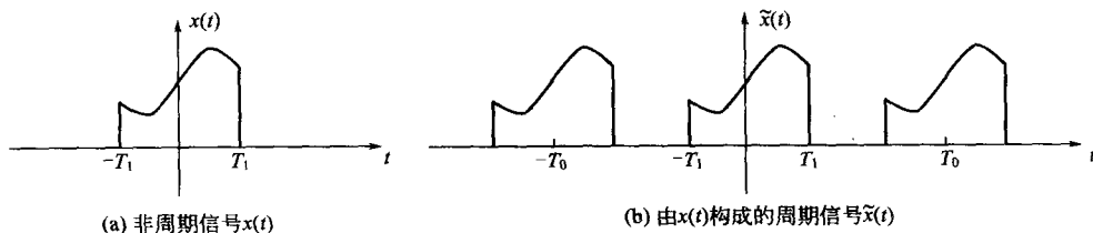
图 3-10 非周期信号的周期延拓
