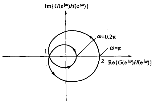
图 8-40 例 8-16 的奈奎斯特图
