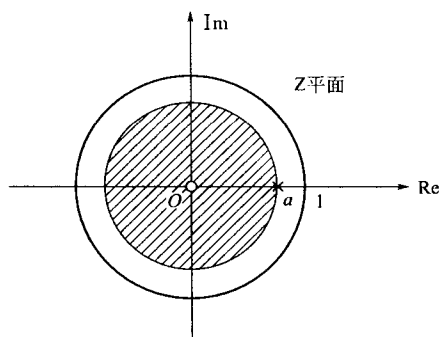
图 7-2 当 0 < a < 1 时, 例 7-2 的零极点和收敛域 (阴影区)
