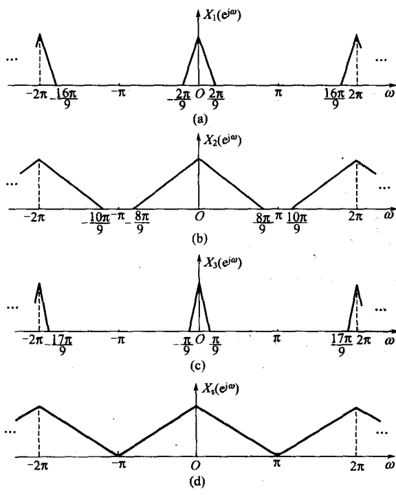
图 5-22 例 5-1 的有关频谱
