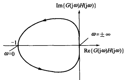
图 8-39 例 8-15 的奈奎斯特图
