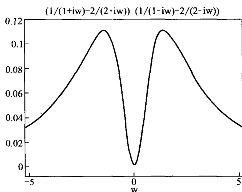
图 3-23 两相加指数信号的能量密度谱
