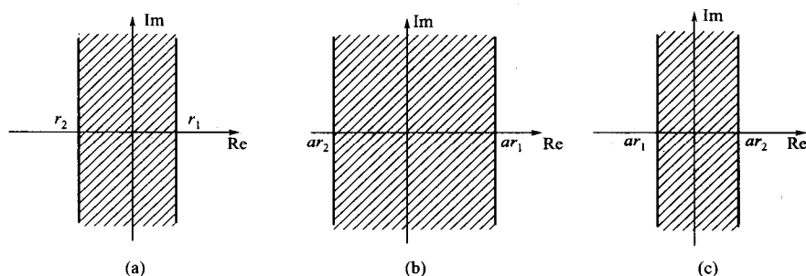
图 6-14 时域尺度变换在 ROC 上的变化
