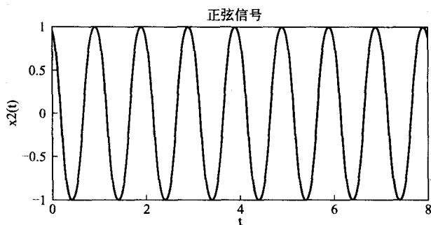
图 1-16 正弦信号波形 (例 1-2 图)
