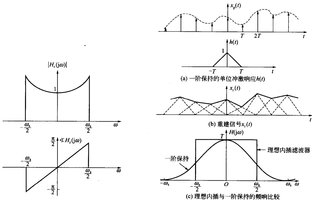
图 5-10 零阶保持输出信号的重建滤波器的模和相位特性
