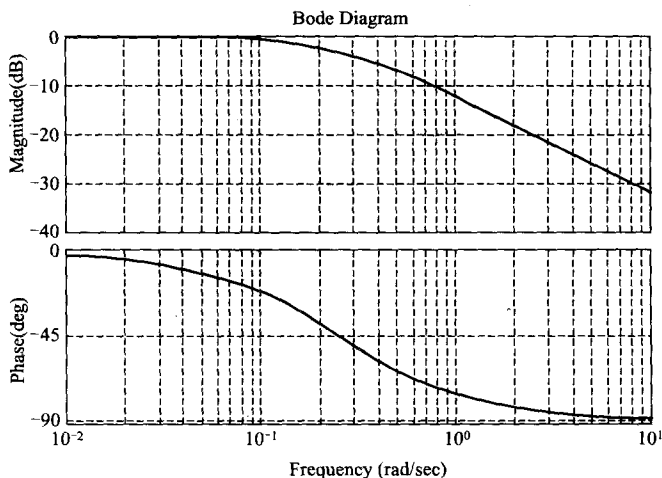
图 8-41 例 8-17 的波特图
