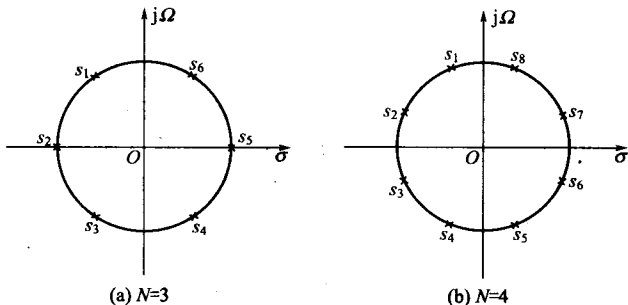
图 8-22 巴特沃思低通滤波器 |H(s)|^2 的极点分布
