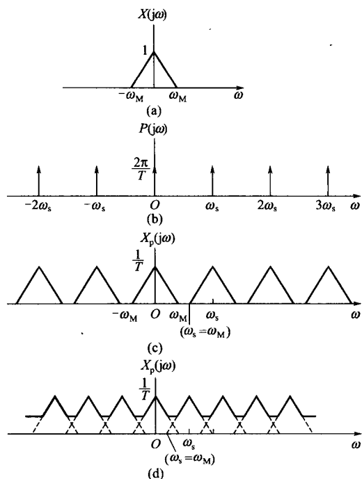
图 5-2 时域采样的各信号的频谱
