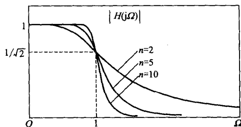
图 8-21 n=2, 5, 10 时的巴特沃思滤波器的幅频特性
