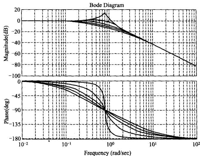
图 8-42 例 8-18 的波特图
