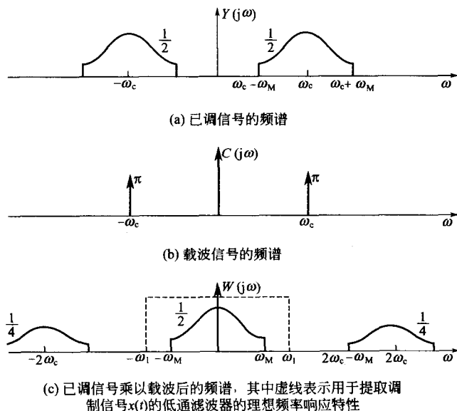
图 5-35 同步解调的频谱说明
