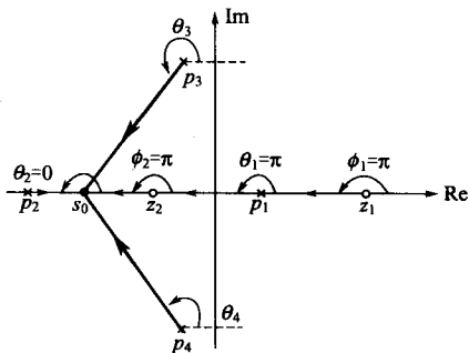
图 8-29 检验实轴上的根轨迹
