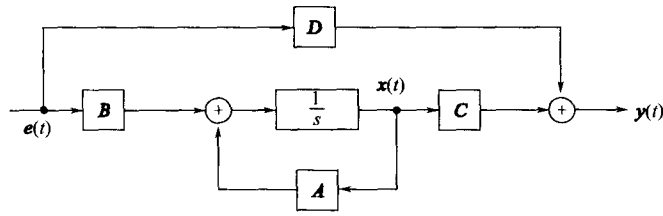
图 9-10 系统状态变量分析示意图
