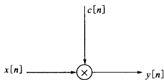
图 5-44 离散时间幅度调制
