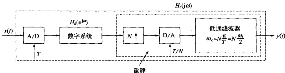
图 5-28 带限连续时间信号的数字化处理
