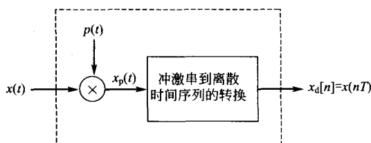
图 5-25 采样系统的等效模型
