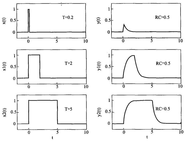
图 3-35 例 3-20 的运行结果: RC 低通网络对矩形脉冲的响应
