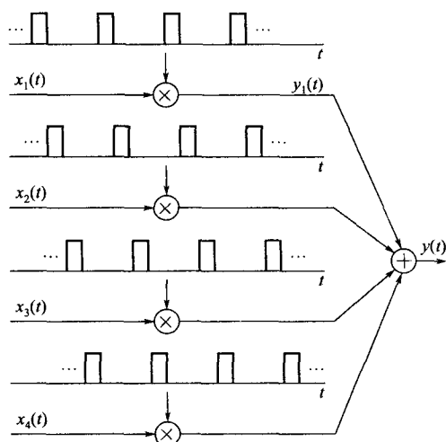
图 5-40 时分复用
