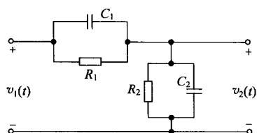
图 3-29 无失真传输系统电路图 (当 R_1 C_1 = R_2 C_2 时)
