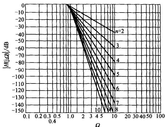
图 8-23 巴特沃思滤波器的幅频特性 (波特图)
