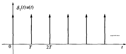
图 6-16 周期重复的冲激信号 \delta_T(t)u(t)
