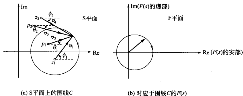
图 8-34 从 S 平面到 F 平面的围线映射
