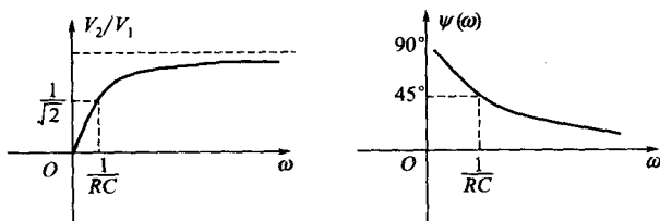
图 6-22 例 6-19 系统的幅频、相频特性
