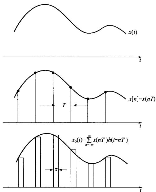
图 5-7 零阶保持
