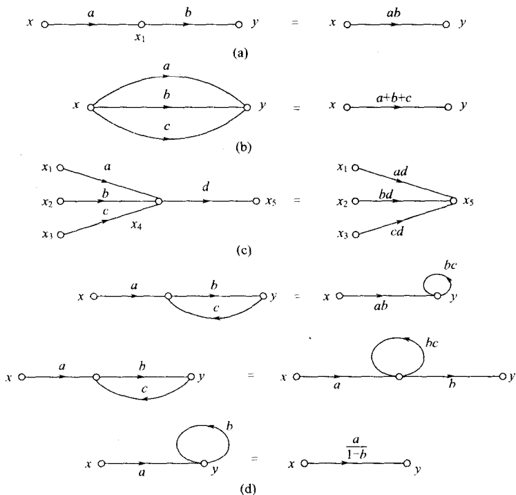
图 9-6 流图的化简规则
