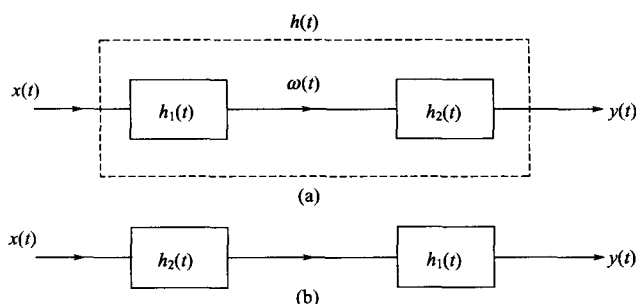
图 2-10 卷积结合律及交换律的系统意义
