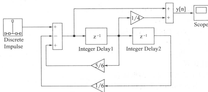
图 2-41 例 2-26 的 Simulink 仿真框图
