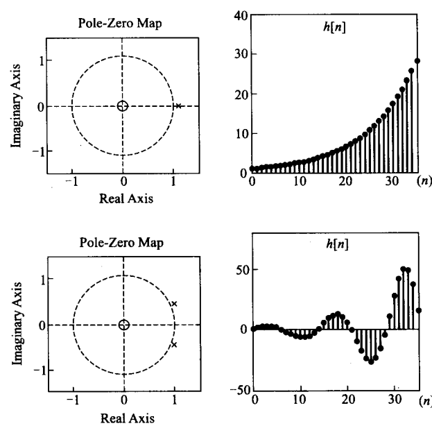
图 8-8 单位圆外的一阶实极点与共轭极点对应的的时间信号
