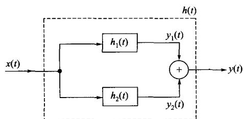
图 2-11 分配律的系统意义
