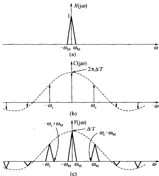
图 5-39 自然采样形式的脉冲幅度调制的频谱说明
