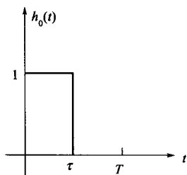
图 5-6 零阶保持重建时, 低通的单位冲激响应
