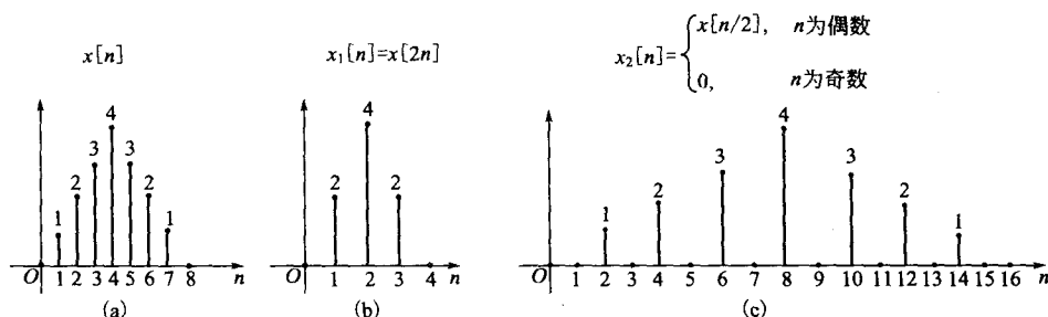
图 1-57 离散时间序列抽取和内插过程
