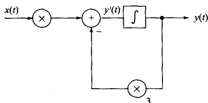
图 6-27 例 6-23 时域模拟框图
