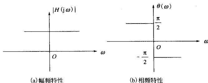
图 5-43 理想的 \frac{\pi}{2} 移相器
