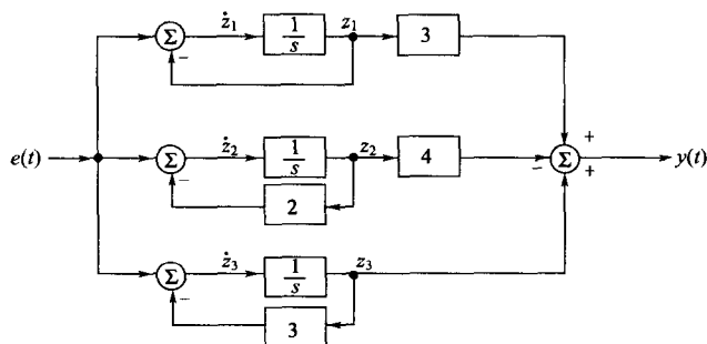
图 9-14 并联实现
