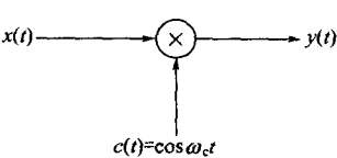
图 5-31 正弦载波的 幅度调制 (DSB)
