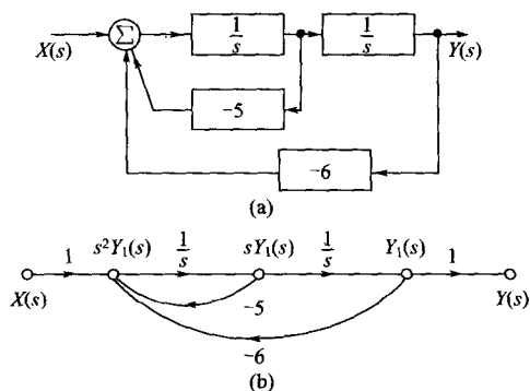
图 9-1 系统的模拟框图和信号流图表示
