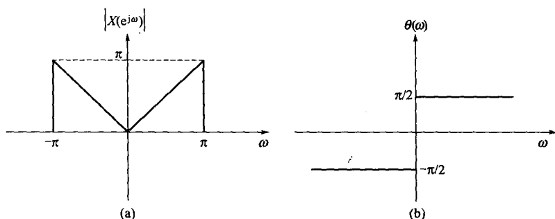
图 4-14 离散时间信号 x[n] 的幅度谱与相位谱
