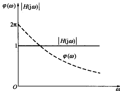
图 8-11 二阶全通系统的频率响应
