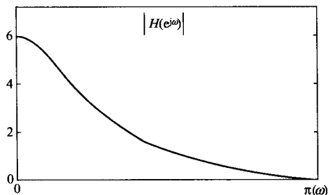
图 4-23 例 4-20 系统的幅度响应
