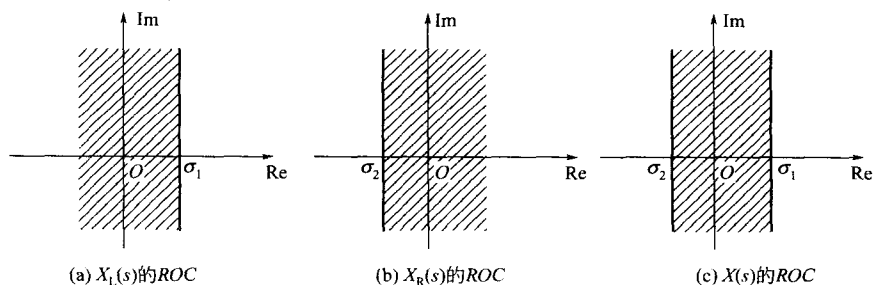
图 6-10 双边信号的拉氏变换收敛域
