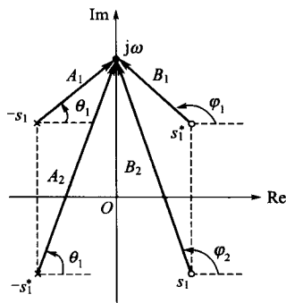
图 8-10 二阶全通系统的零极点矢量图
