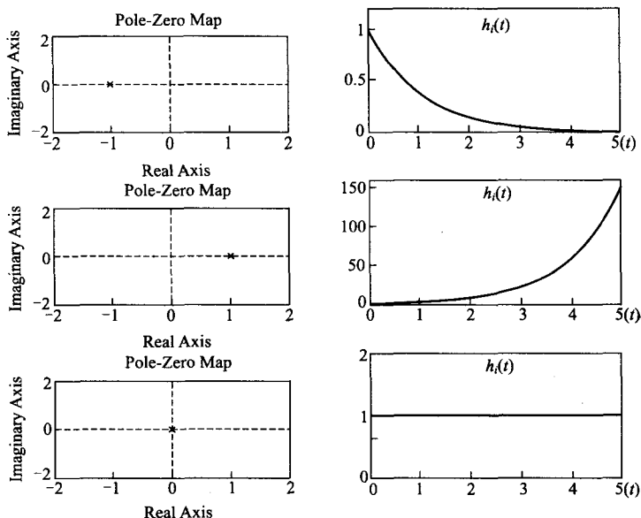
图 8-1 一阶实极点对应的时间函数
