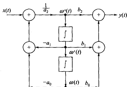
图 2-27 二阶系统的模拟框图
