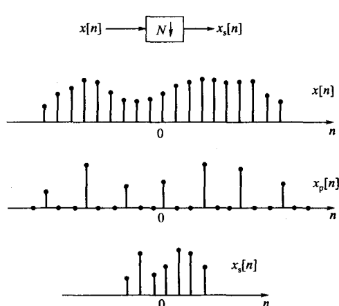
图 5-18 信号的抽取
