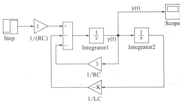
图 2-39 例 2-25 中 LC 并联电路的 Simulink 仿真框图
