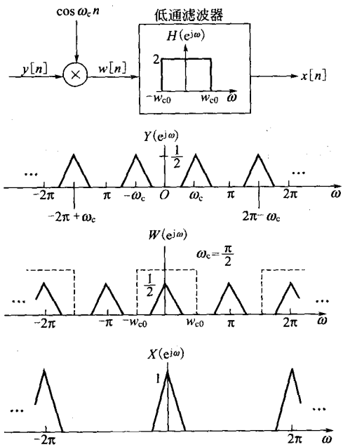
图 5-46 离散时间同步解调及其相关频谱说明 ( \omega_c = \frac{\pi}{2} )
