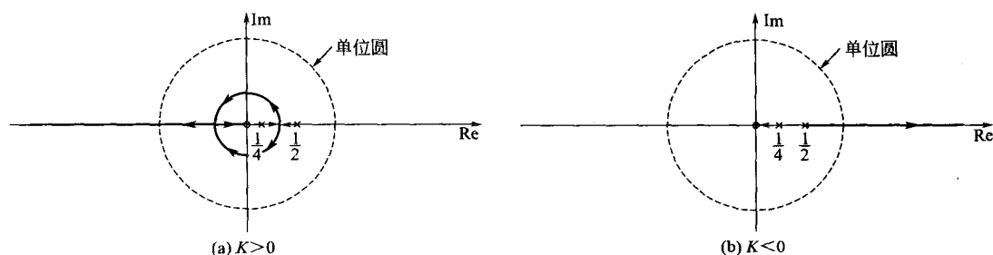
图 8-32 例 8-11 的根轨迹
