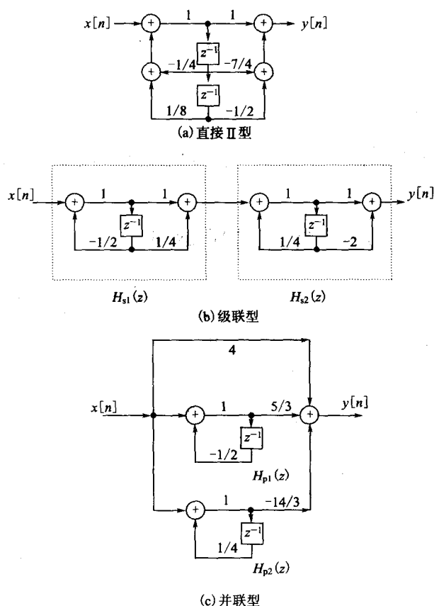
图 7-12 例 7-25 系统的 Z 域框图表示
