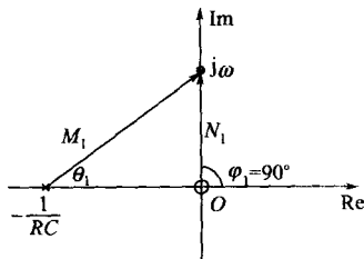
图 6-21 高通滤波器的零极点图
