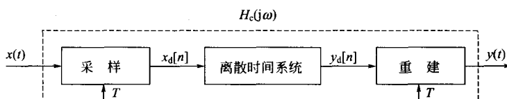
图 5-24 连续时间信号的离散时间处理，其中 x_d[n] = x(nT) , y_d[n] = y(nT)
