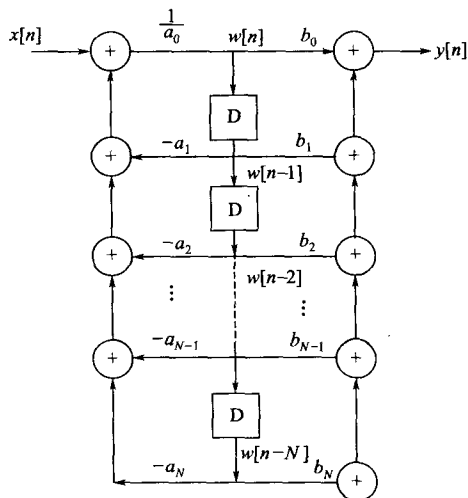
图 2-31 N 阶离散系统的模拟框图
