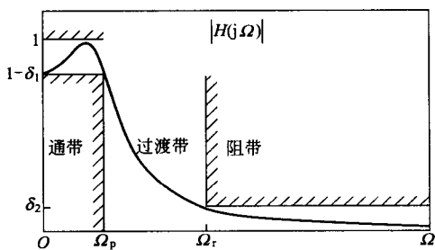
图 8-19 低通滤波器的幅频特性
