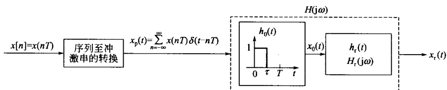
图 5-9 零阶保持的恢复系统
