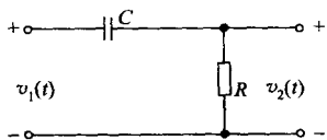
图 6-20 RC 高通滤波器
