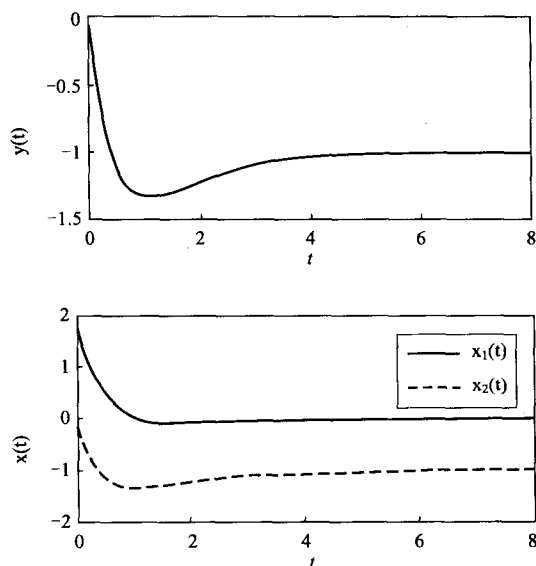
图 9-21 例 9-27 输出变量和状态变量响应曲线
