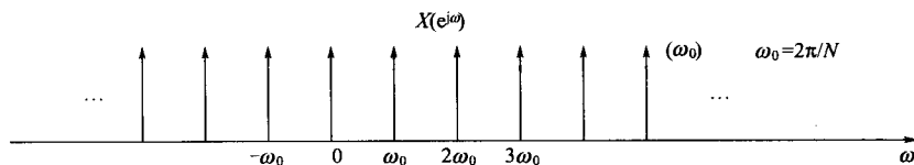
(b) 离散时间周期冲激串的频谱
