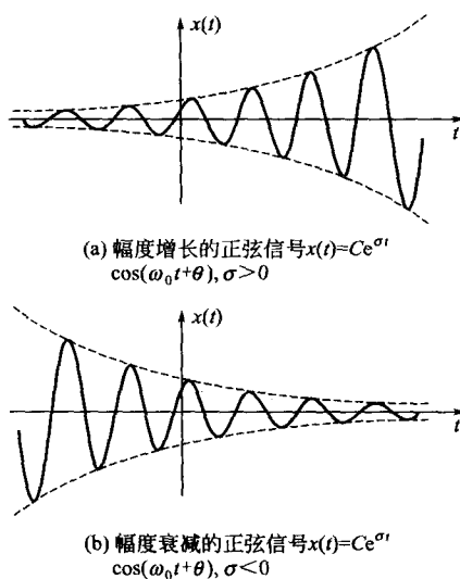
图 1-14 振幅呈指数增长或指数衰减的正弦信号
