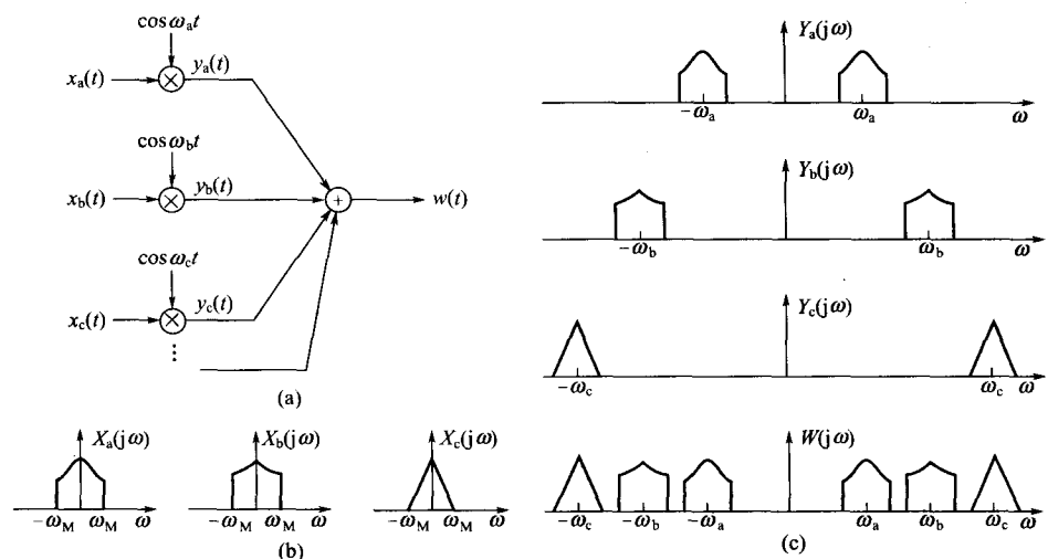
图 5-36 频分多路复用
