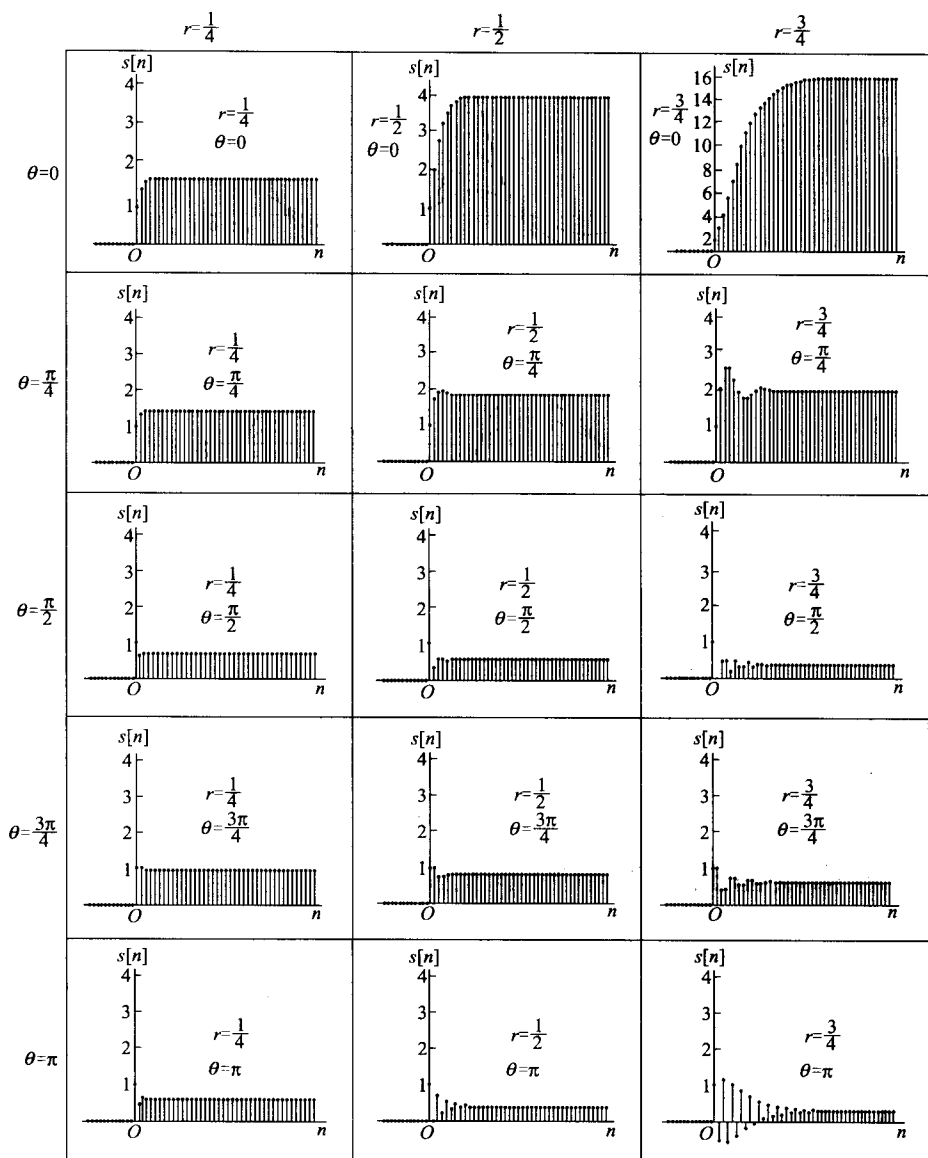
图 8-17 由方程式(8-65)表示的二阶系统的单位阶跃响应
