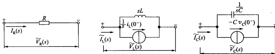
图 6-24 S 域元件模型 (节点分析)
