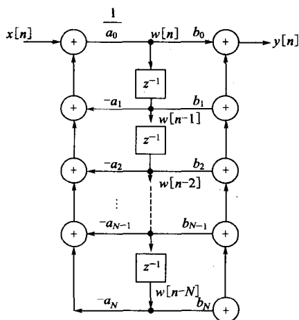
图 7-11 N 阶离散系统的 Z 域直接 II 型模拟框图
