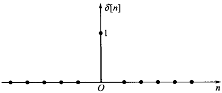
图 1-34 离散单位脉冲序列 \delta[n]
