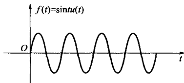
图 1-20 \sin tu(t) 波形
