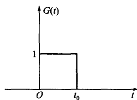
图 1-21 矩形脉冲
