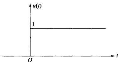
图 1-17 单位阶跃信号
