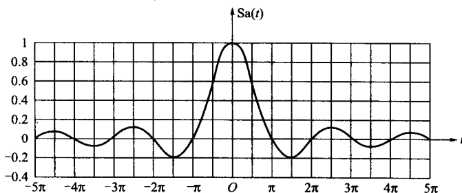
图 1-31 Sa(t) 波形
