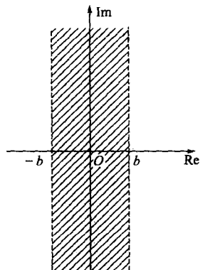
图 6-3 例 6-2 中信号的收敛域
