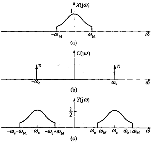
图 5-33 DSB 调制的频谱说明
