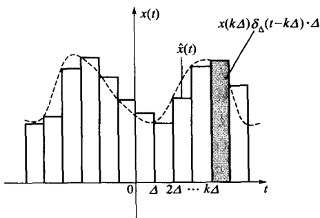
图 2-4 用矩形脉冲逼近 x(t)
