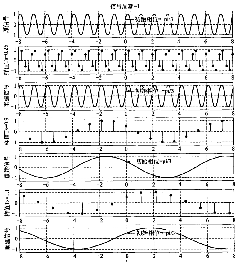
图 5-14 欠采样的效果
