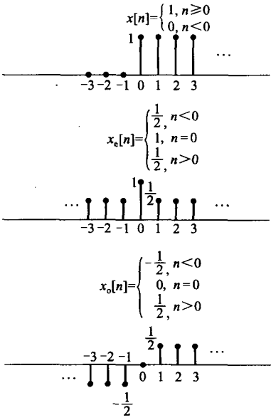
图 1-7 离散时间信号分解
