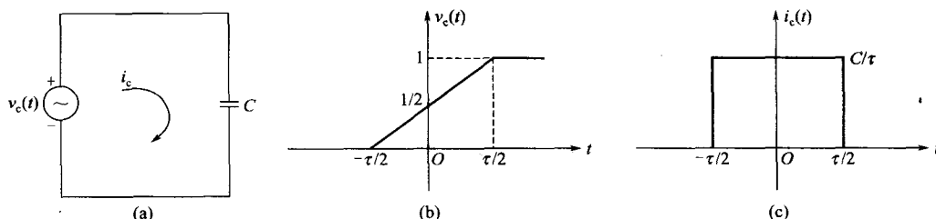
图 1-28 \delta(t) 信号的物理意义
