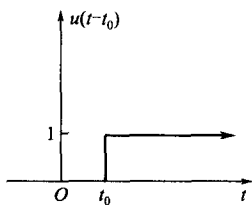
图 1-19 延迟的单位阶跃信号
