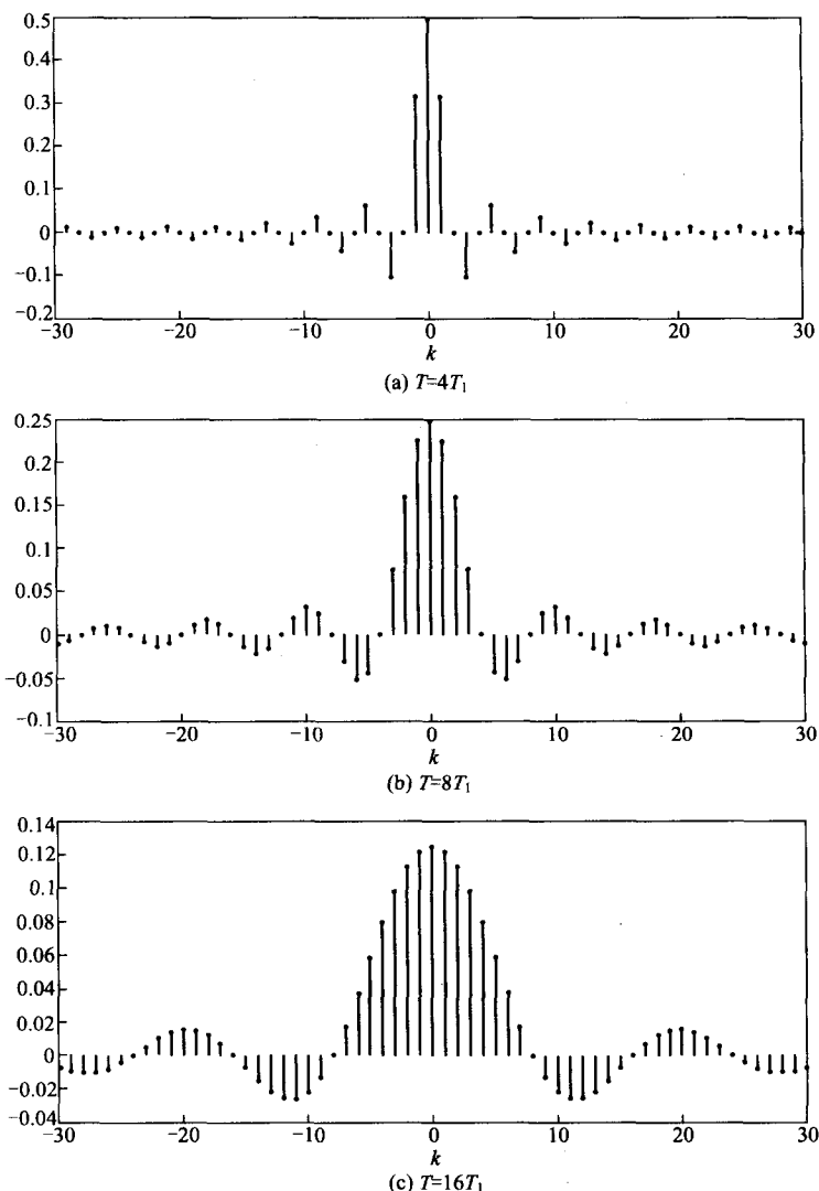
图 3-3 对于 T_1 固定和几个不同的 T 值时, 周期方波傅里叶级数系数 a_k 的图
