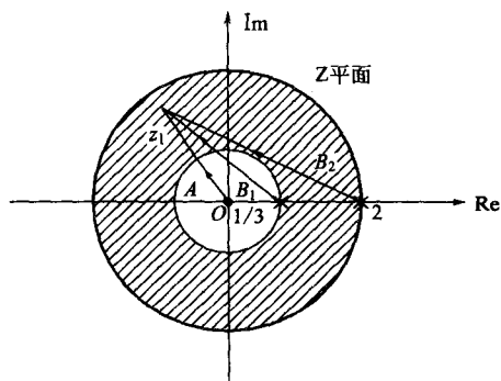
图 7-7 零极点矢量
