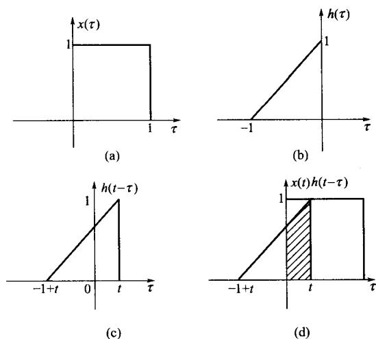
图 2-7 卷积 x(t) * h(t) 的图示
