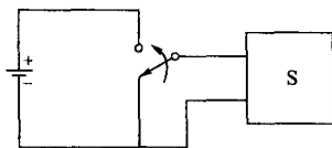
图 1-18 单位阶跃信号的物理意义
