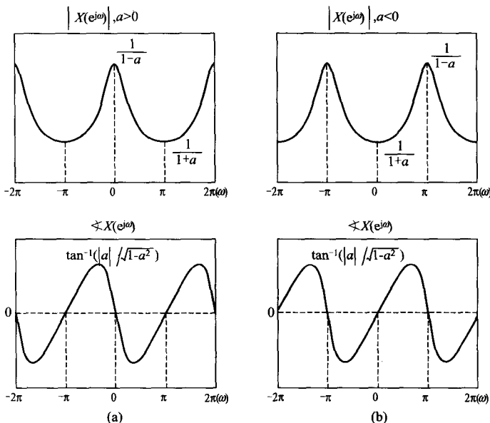
图 4-5 单边指数衰减信号的幅度谱与相位谱
