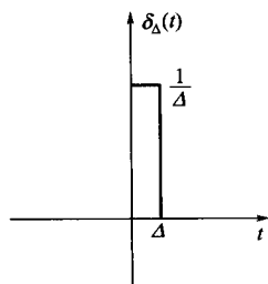
图 2-2 \delta_{\Delta}(t) 波形
