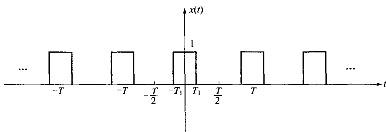
图 3-2 周期方波
