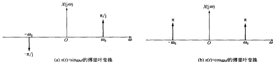
图 3-19 正弦和余弦信号的频谱
