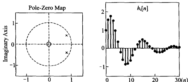
图 8-4 单位圆内一阶共轭复极点及其对应的时间信号
