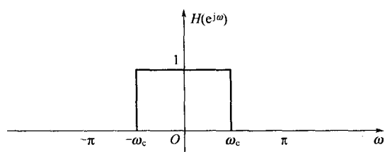
图 4-18 离散时间理想低通滤波器的频率响应
