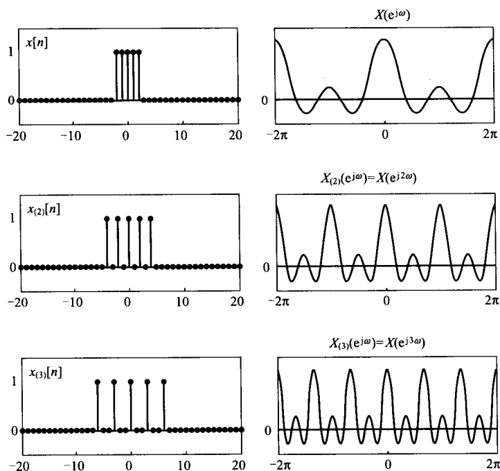
图 4-13 离散时间情况下时域与频域的反向关系: 当 k 增加时, x_{(k)}[n] 在时域上拉开, 而其傅里叶变换则在频域上压缩
