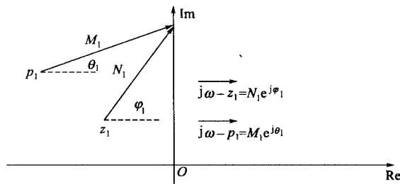
图 6-19 零点、极点矢量
