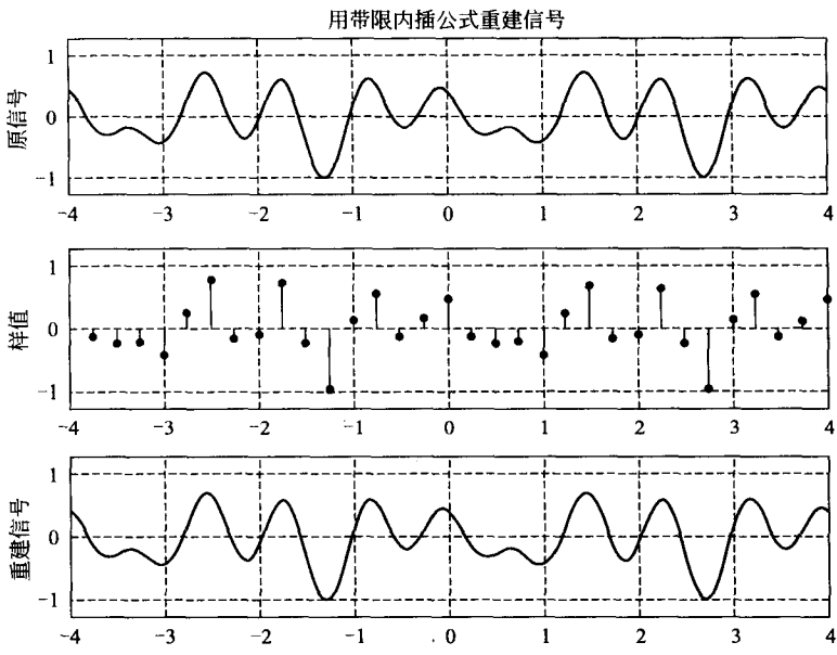
图 5-5 用带限内插公式重建信号
