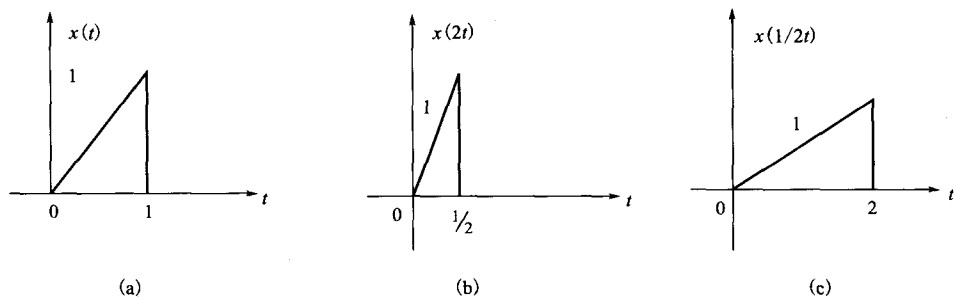
图 1-54 信号的尺度变换
