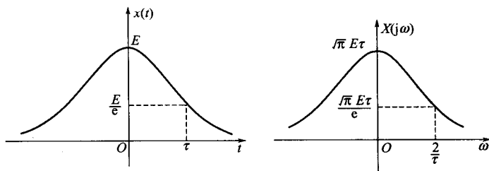
图 3-16 高斯脉冲信号的波形及频谱
