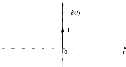
图 1-26 冲激信号 \delta(t)
