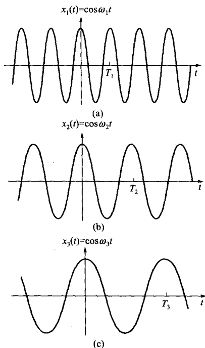
图 1-13 连续时间正弦信号基波频率与周期之间的关系
