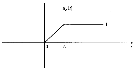
图 1-24 斜平信号 u_{\Delta}(t)
