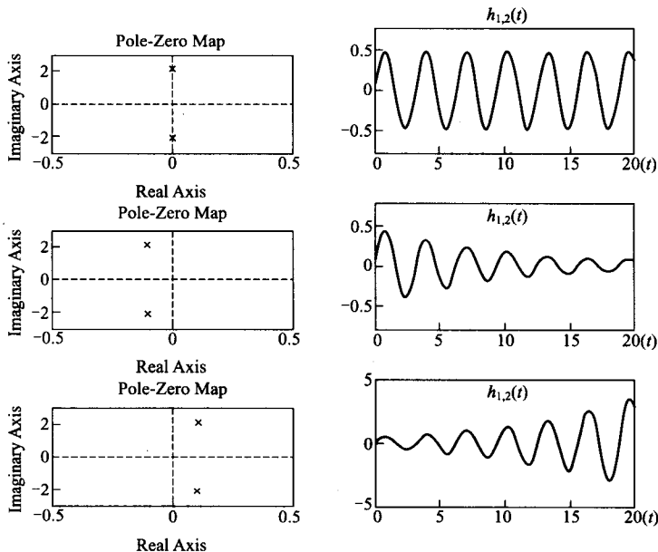
图 8-2 一阶共轭复极点对应的的时间函数
