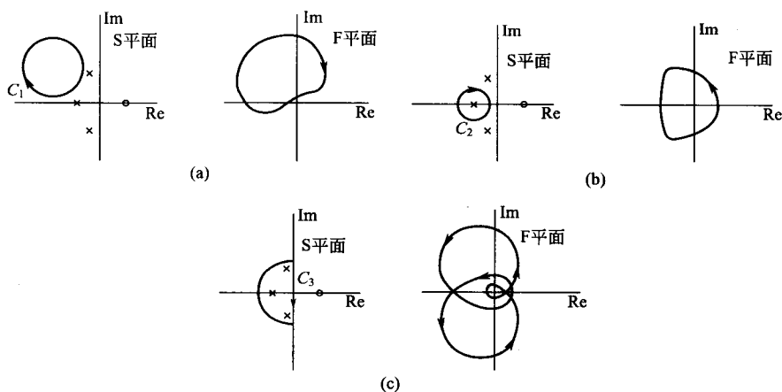
图 8-35 例 8-13 围线映射图
