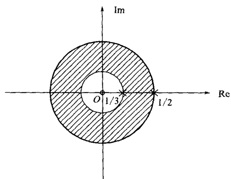
图 7-6 例 7-5 的 ROC
