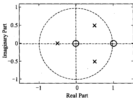
图 7-15 例 7-31 零极点图
