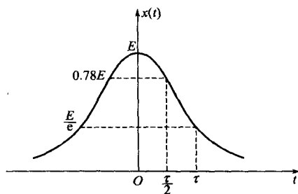
图 1-33 钟形脉冲信号
