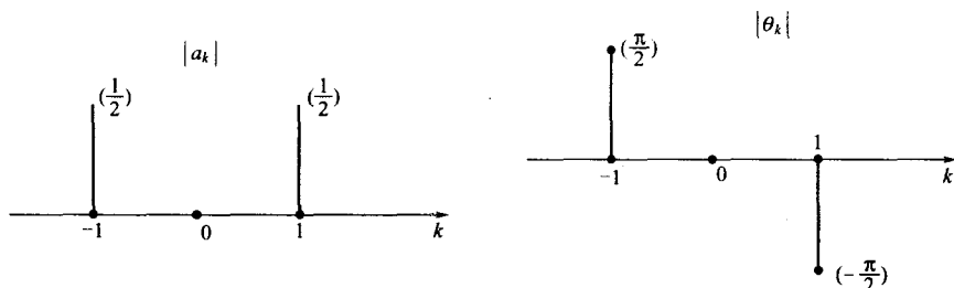
图 3-1 \sin\omega_0 t 信号的傅里叶级数系数的幅度和相位
