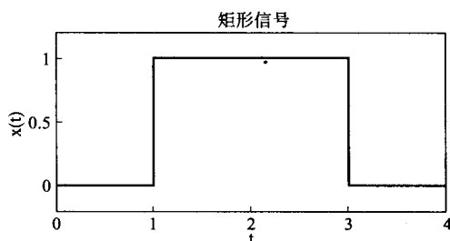
图 1-22 矩形脉冲信号 (例 1-3 图)
