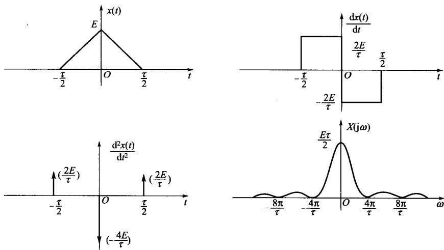
图 3-21 三角脉冲信号的波形和频谱
