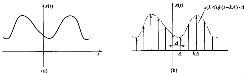
图 2-1 用移位冲激函数逼近 x(t)
