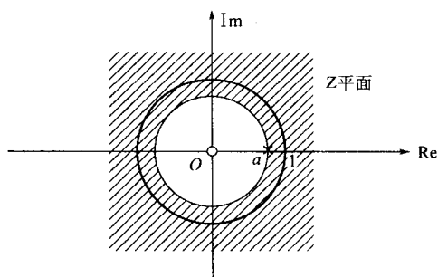
图 7-1 当 0 < a < 1 时, 例 7-1 的零极点和收敛域 (阴影区)
