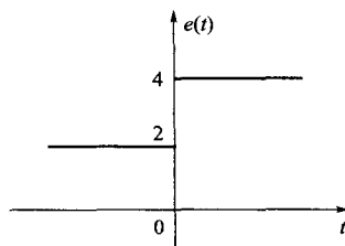
图 2-23 例 2-14 的输入信号波形
