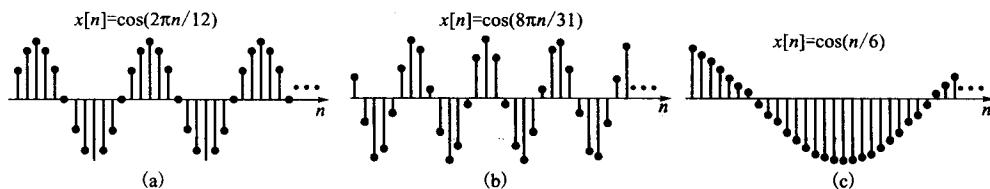
图 1-42 周期与非周期序列
