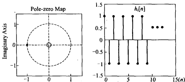
图 8-6 极点为 -1 及其对应的时间信号
