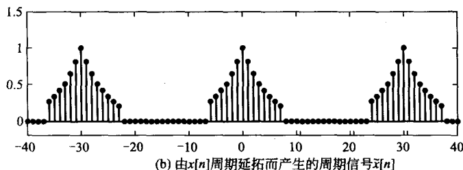
图 4-3 离散时间的有限长信号与周期信号
