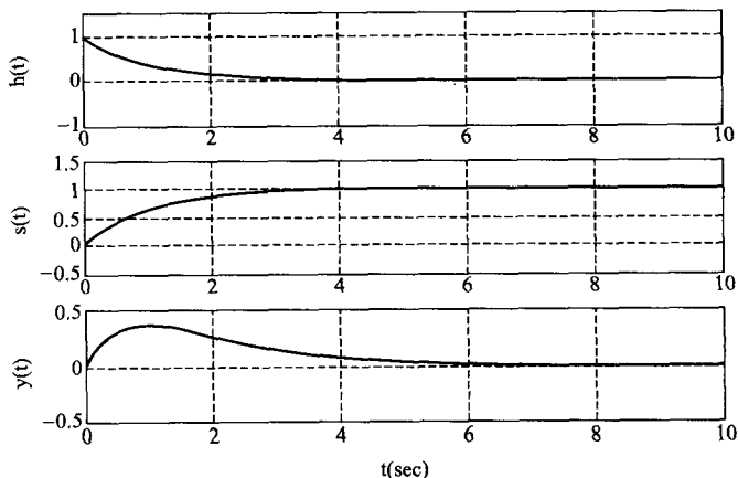
图 2-32 例 2-20 的运行结果图
