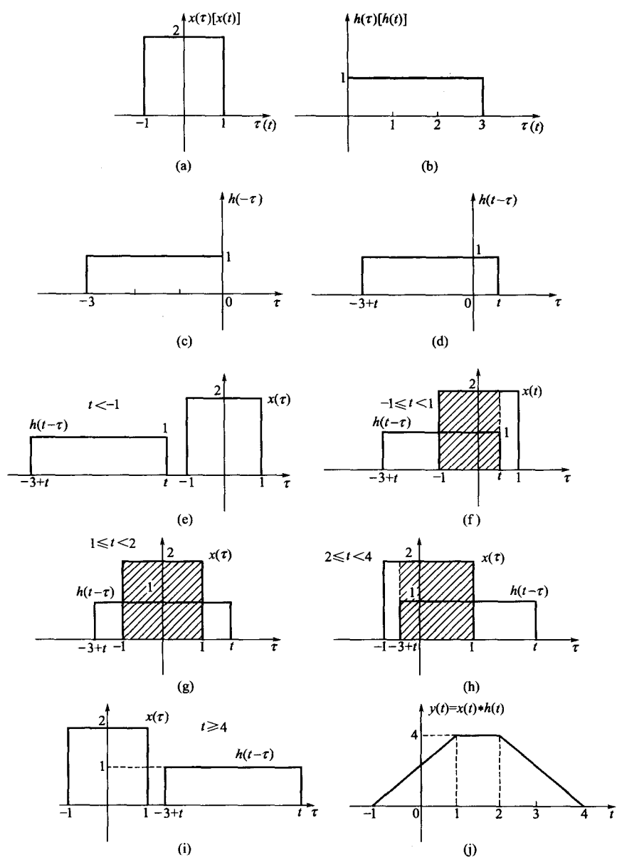
图 2-8 例 2-2 卷积的图解示意图
