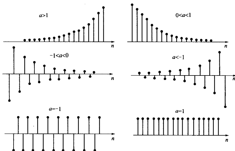
图 1-41 实指数序列
