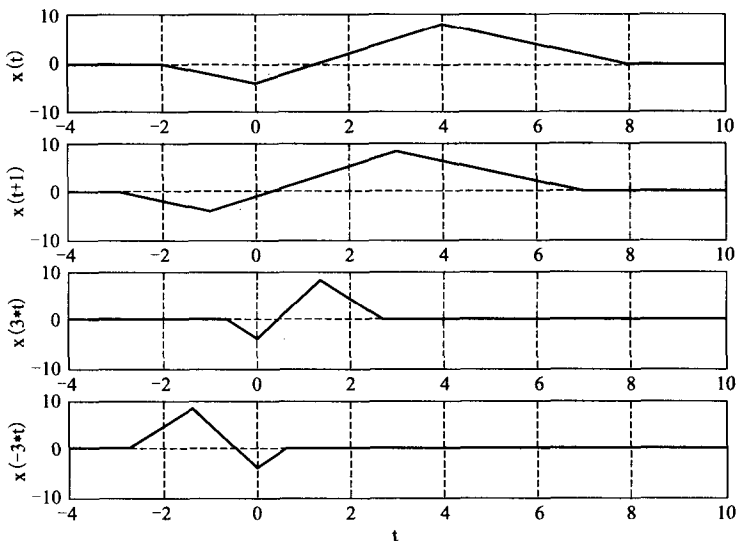
图 1-56 变换函数的波形 (例 1-11 图)
