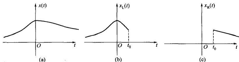
图 6-9 双边信号
