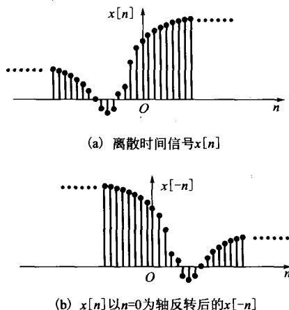
图 1-53 离散信号的反褶
