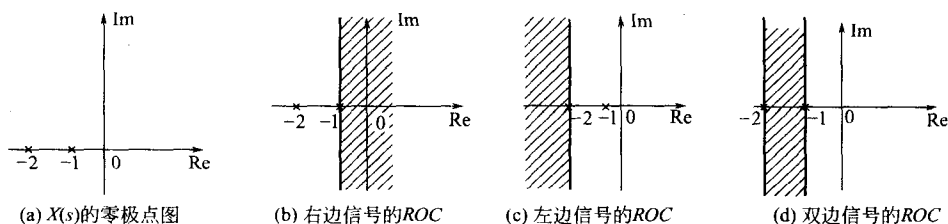
图 6-11 例 6-4 信号拉氏变换 X(s) 的收敛域
