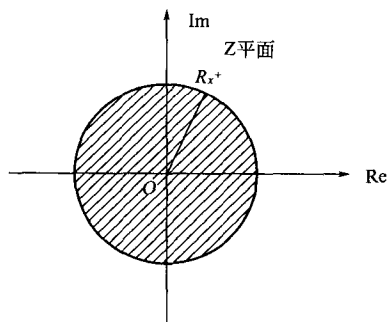
图 7-4 左边序列的 ROC
