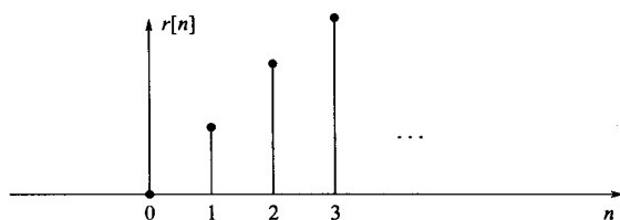
图 1-39 单位斜坡序列 r[n] 的波形
