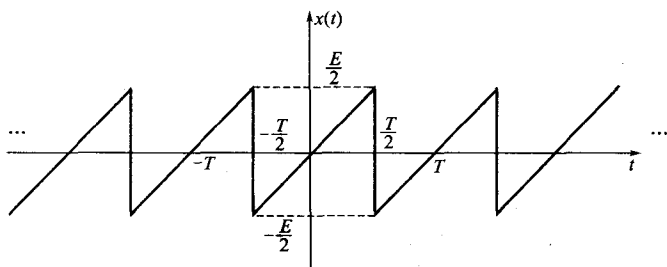
图 3-4 周期锯齿脉冲信号的波形
