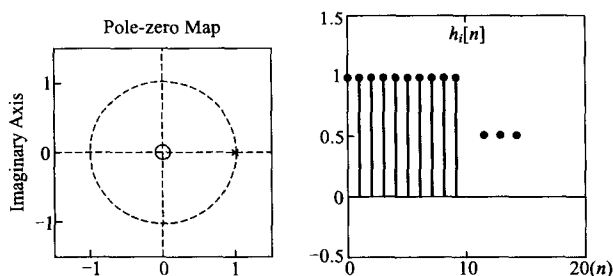
图 8-5 极点为 +1 及其对应的时间信号
