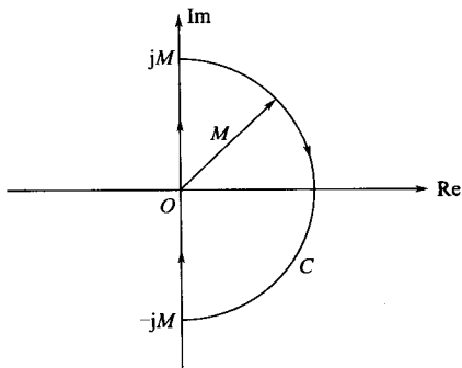
图 8-36 包括右半平面的半圆闭合围线, 当 M \rightarrow \infty 时, 该围线包括了整个右半平面
