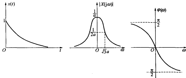
图 3-11 单边指数信号的波形及频谱
