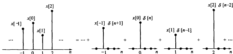
图 2-17 一个离散时间信号分解为一组加权的移位脉冲之和
