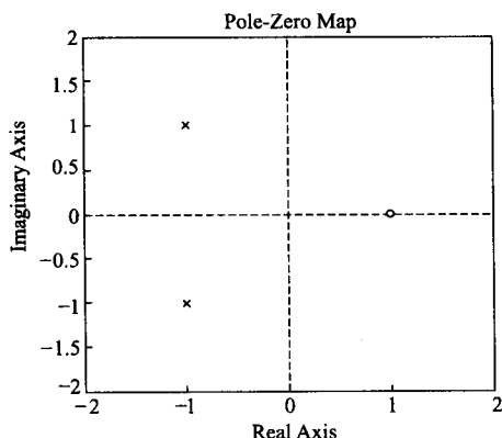
图 6-31 例 6-28 零极点图
