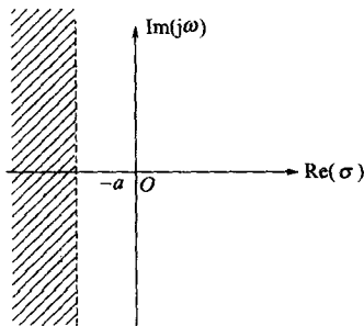
图 6-2 X_2(s) 的收敛域
