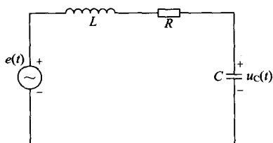
图 8-13 RLC 串联回路
