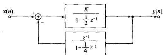
图 8-31 例 8-11 离散时间反馈系统
