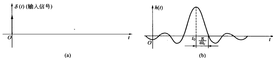
图 3-31 理想低通滤波器的冲激响应
