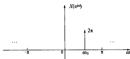
图 4-9 x[n] = e^{j\omega_0 n} 的频谱 ( 0 < \omega_0 < \pi )
