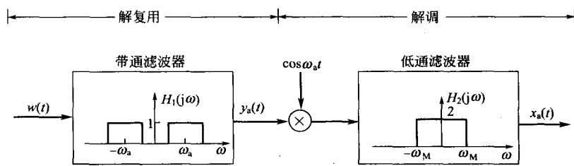
图 5-37 某一路频分复用信号的解复与解调
