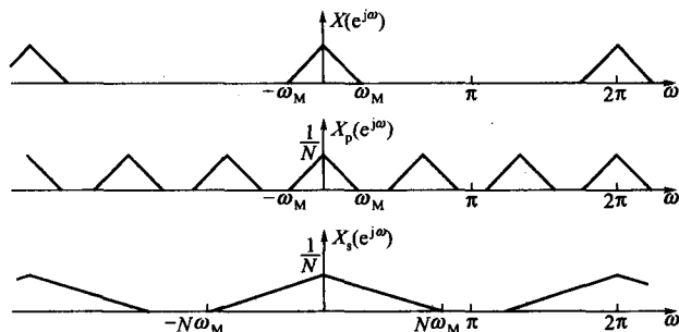
图 5-19 抽取的频域关系
