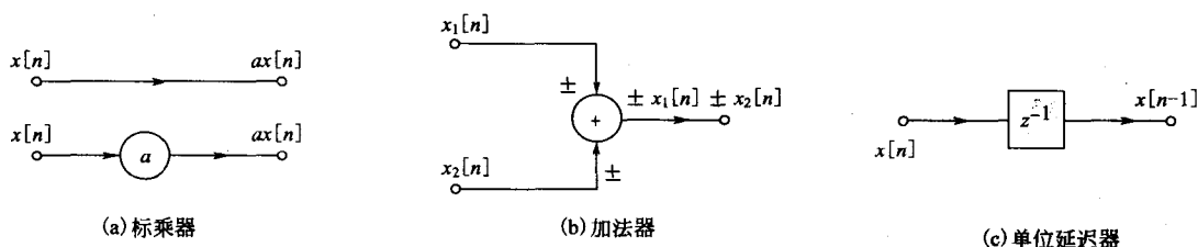
图 7-9 离散系统的三个基本运算单元
