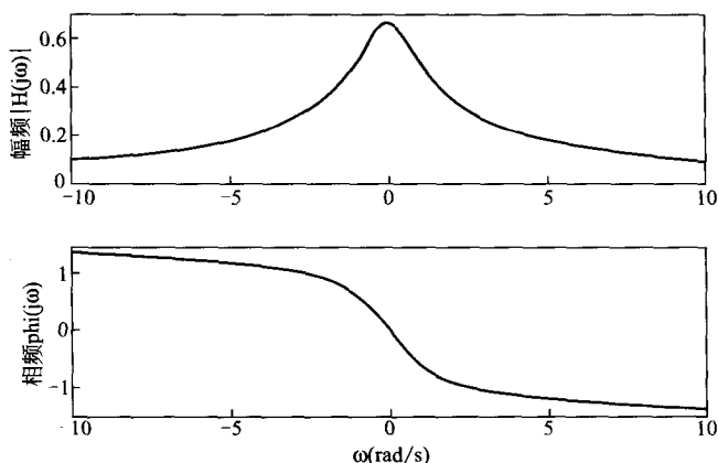
图 3-25 例 3-17 频率响应的幅频特性和相频特性
