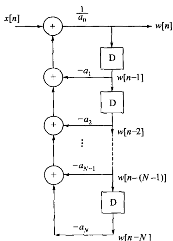
图 2-30 式(2-99) 所描述离散时间系统的模拟框图
