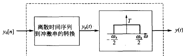
图 5-26 重建系统的等效模型
