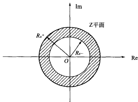
图 7-5 双边序列的 ROC
