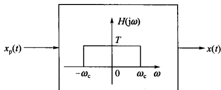
图 5-3 用于恢复的低通滤波器
