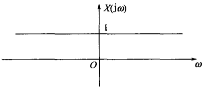
图 3-13 单位冲激信号的频谱
