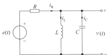
图 2-37 例 2-25 所讨论的 LC 并联电路
