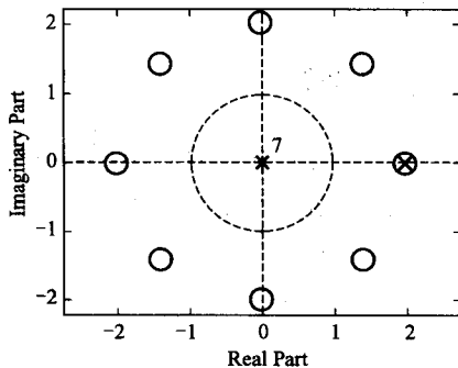
图 7-14 例 7-30 零极点图
